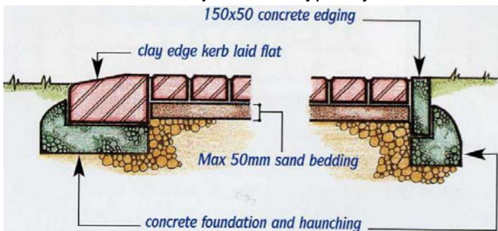
Edge restraints
